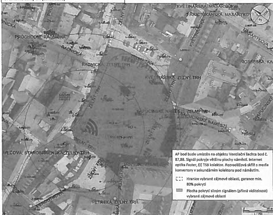
Příloha č. 1: Mapa pokrytí signálem WiFi
