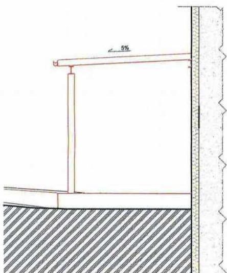
PRAVÝ POHLED NA STŘÍŠKU
