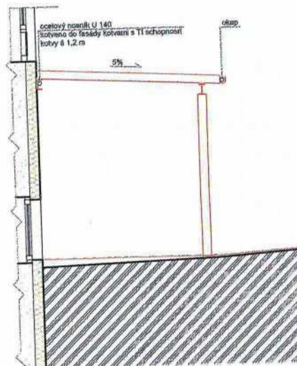
LEVÝ POHLED NA STŘÍŠKU
