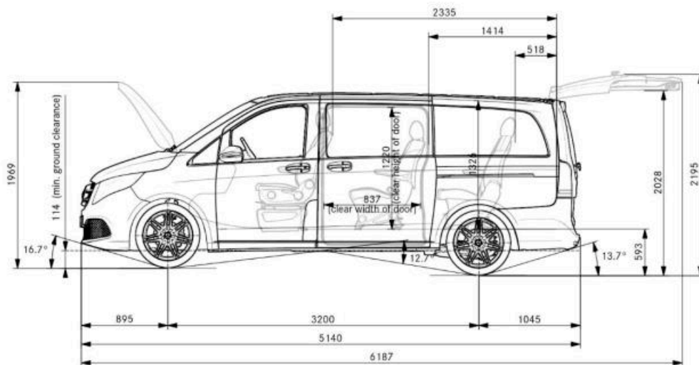
Rozměry podléhají toleranci +/- 3%
