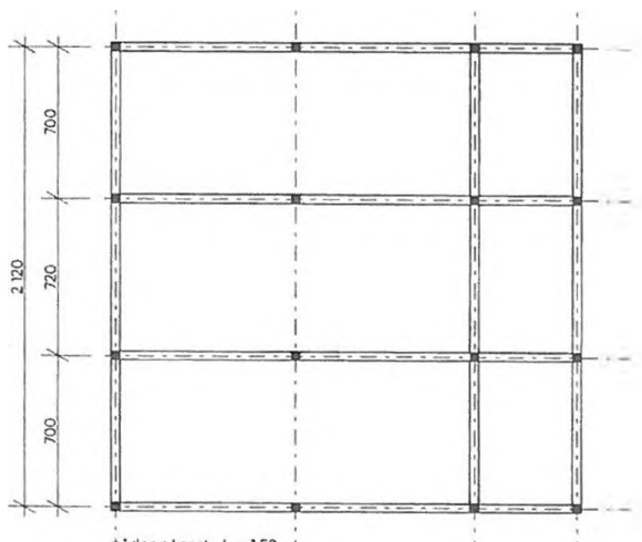
půdorys konstrukce 1:50
