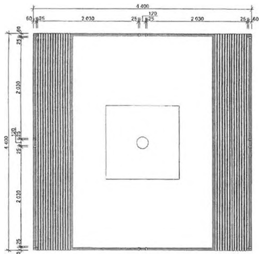
půdorys obkladu 1:50
