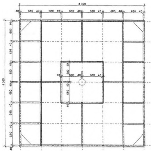
půdorys ječlové konstrukce + oplechování 1:50
