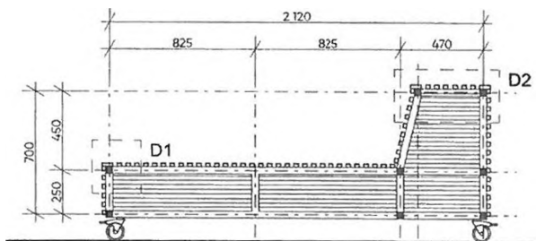
řez konstrukce 1:50
