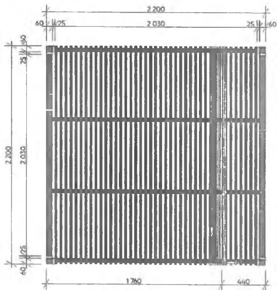
půdorys obložení 1:50
