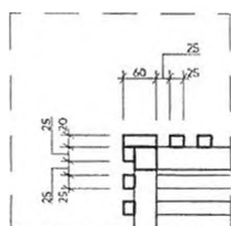
detail obkladu 1:10
