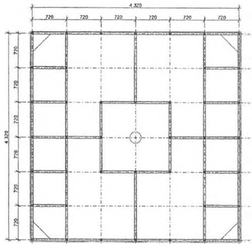
půdorys ječlové konstrukce 1:50
