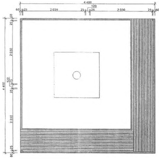
půdorys obkladu 1:50
