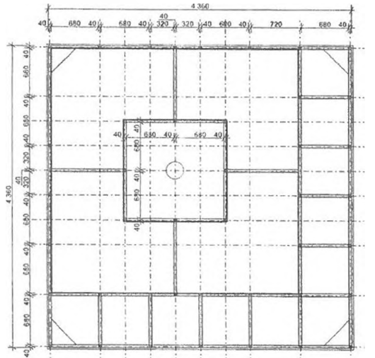
půdorys jeklové konstrukce + oplechování 1:50
