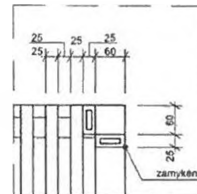
detail napojení lavic v rohu sedací části květináče 1:10
