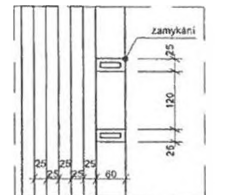
detail napojení lavic na stěnu sedací části květináče 1:10
