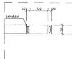
detail napojení lavic na stěnu květináče 1:10
