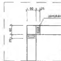
detail napojení lavic v rohu květináče 1:10
