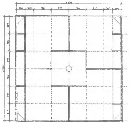
půdorys jeklové konstrukce 1:50
