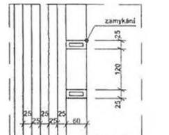
detail napojení lavic na stěnu sedací části květináče 1:10
