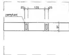
detail napojení lavic na stěnu květináče 1:10
