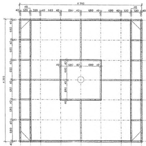
půdorys jeklové konstrukce + oplechování 1:50
