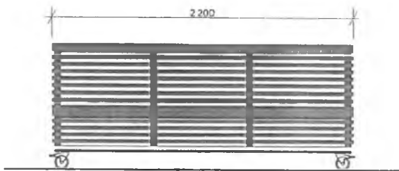
čelní pohled 1:50
