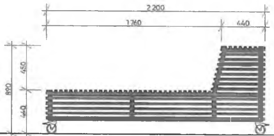
boční pohled 1:50
