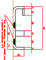
Vodící koleje s pojítkou na podtluk
