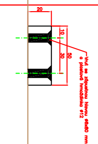
Hlavičky koleje na podtluk
