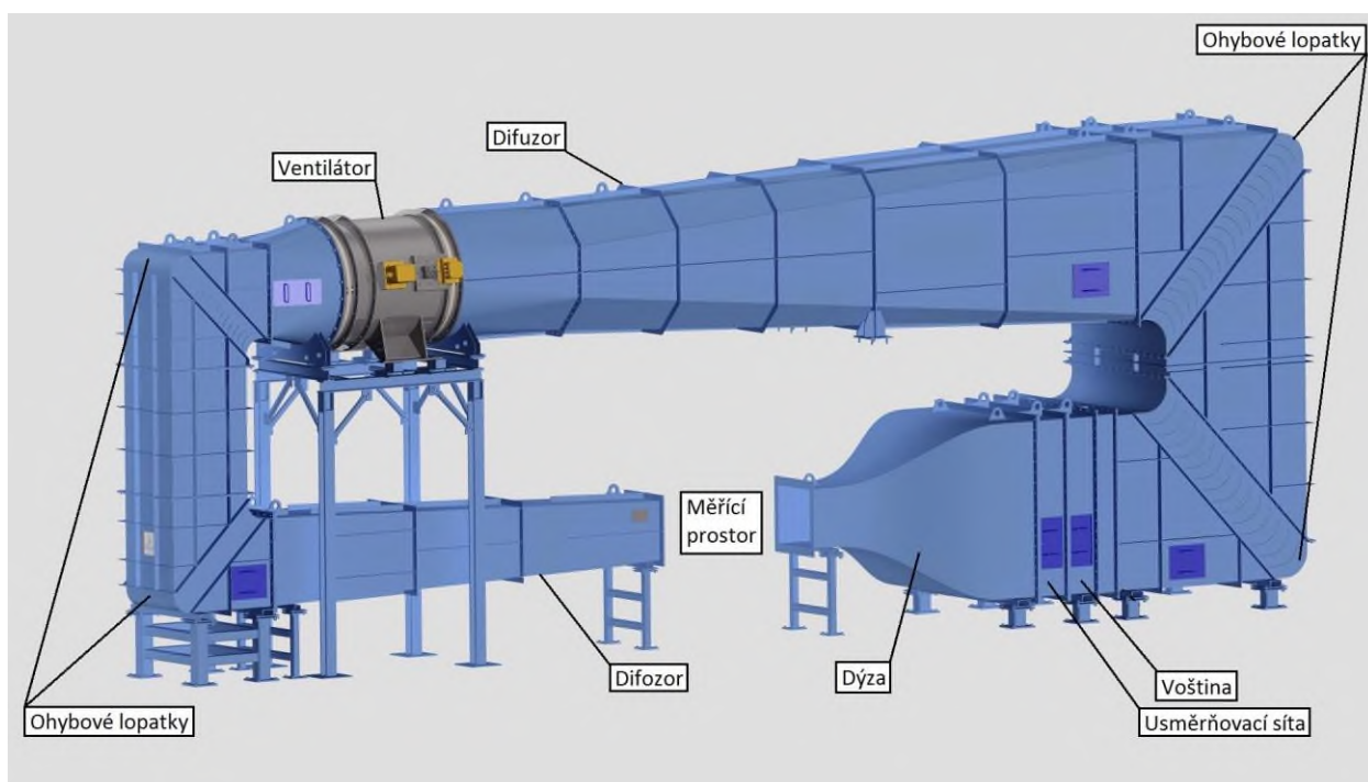
Aerodynamický (větrný) tunel - hlavní části tunelu
