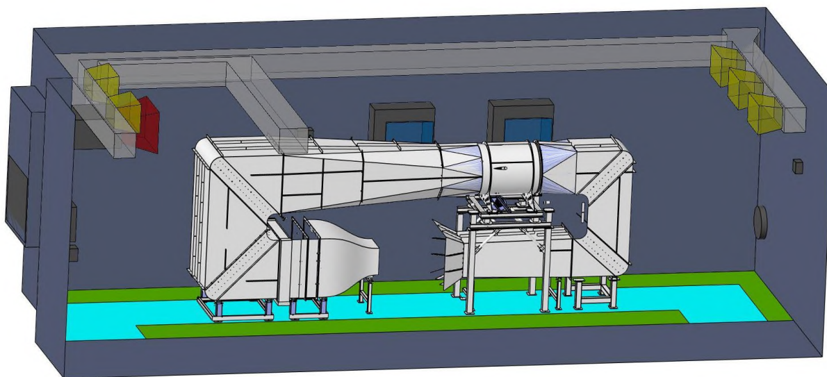
Předběžný 3D model aerodynamického tunelu umístěný v laboratoři s hlavními částmi
