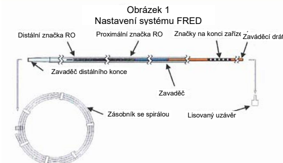
Obrázek 2 Názvosloví systémových značek FRED
