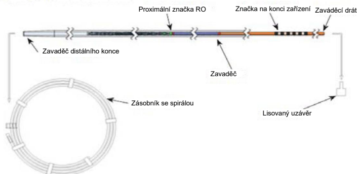
Obrázek 2 Návosloví systémových značek FRED Jr.
