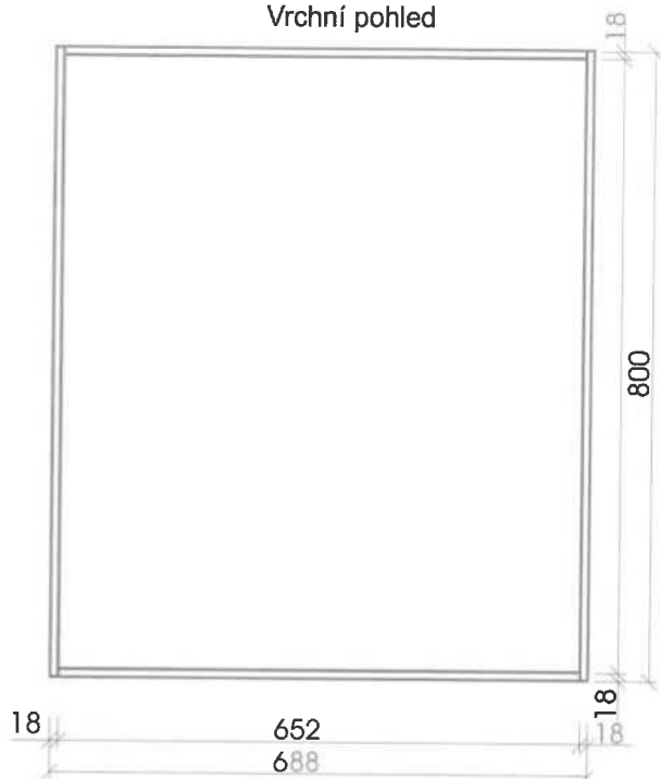
Vrchní pohled
