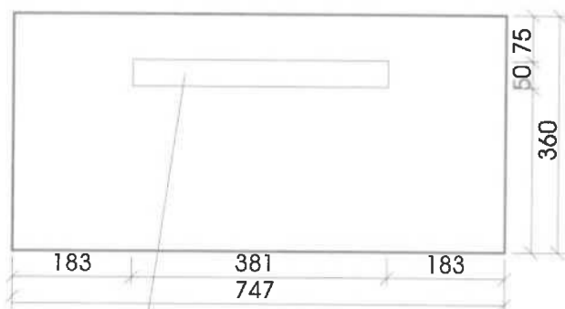
Čelo šuplíku
