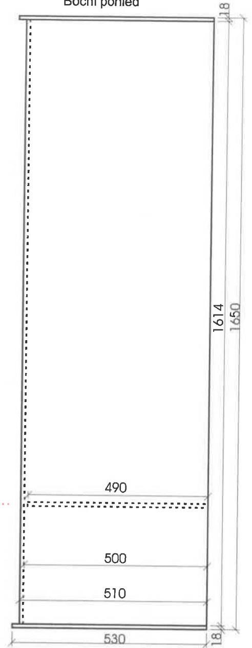
Boční pohled
