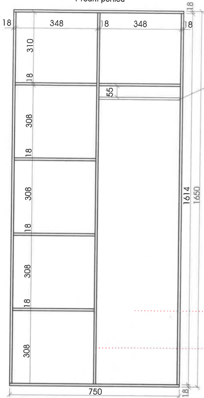
Přední pohled
