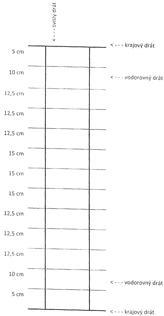
Příloha 1.: Schematické znázornění rozestupů drátů
