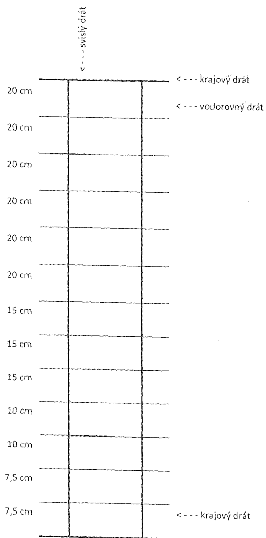
Příloha 1.: Schematické znázornění rozestupů drátů
