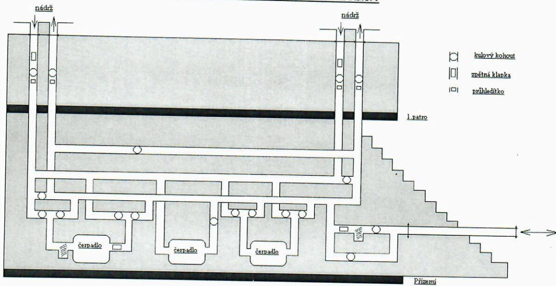
Schéma technologie BLPH č. 58 Pardubice
