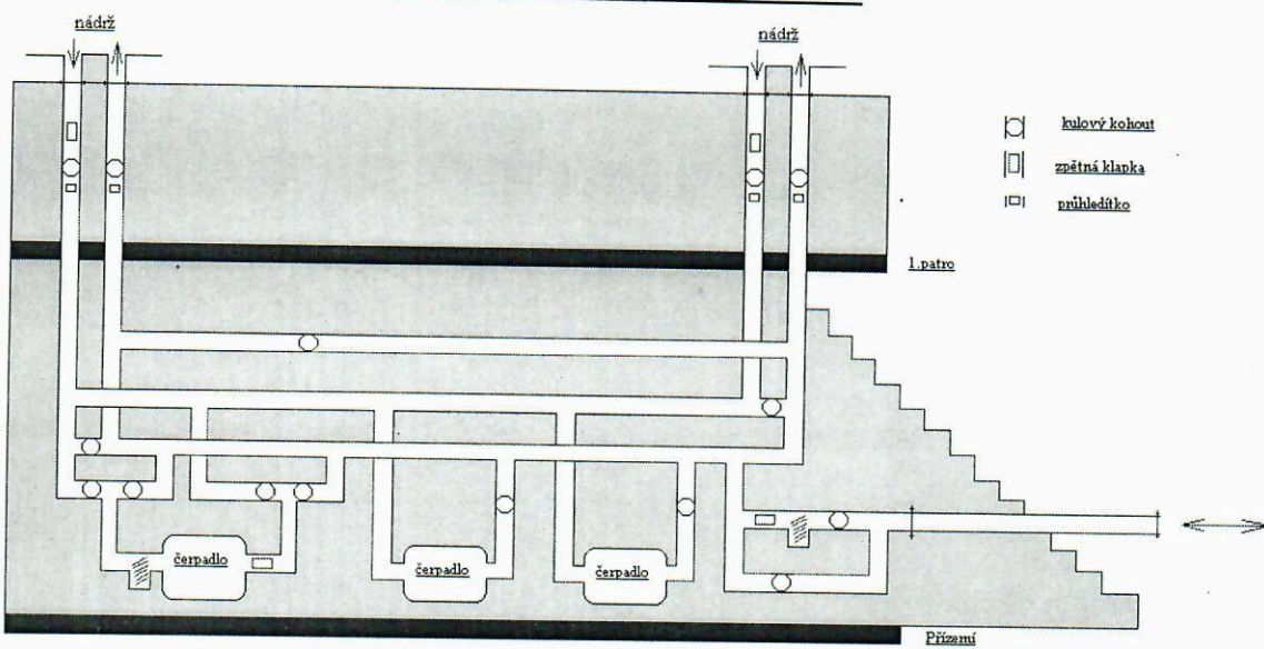
Schéma technologie BLPH č. 59 Pardubice
