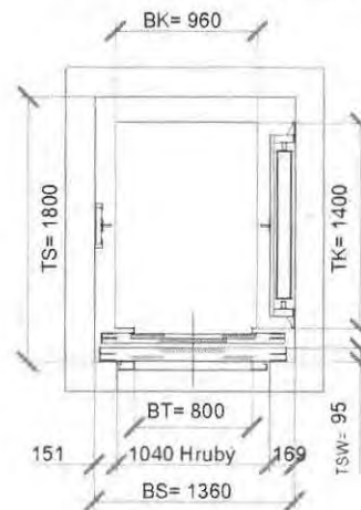
Půdorys šachty 1:50
