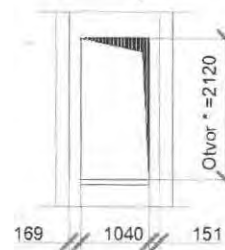
Stavební otvory dveří 1:100 Pohled ze šachty
