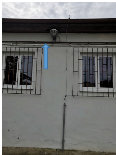
8. Oprava osvětlení – výbojkové lampy 3 kusy na plášti SO č. 040 oprava (výměna) výbojkových světel.
