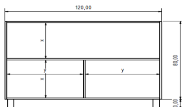
ČELNÍ POHLED - základní kus - spodní police
