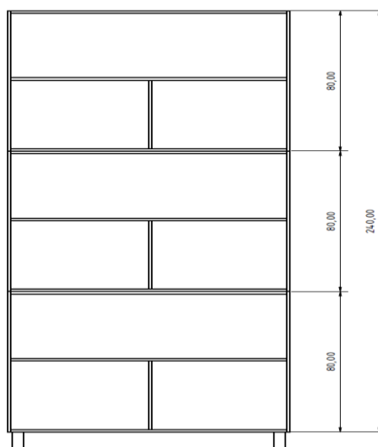
ČELNÍ POHLED - celková sestava
