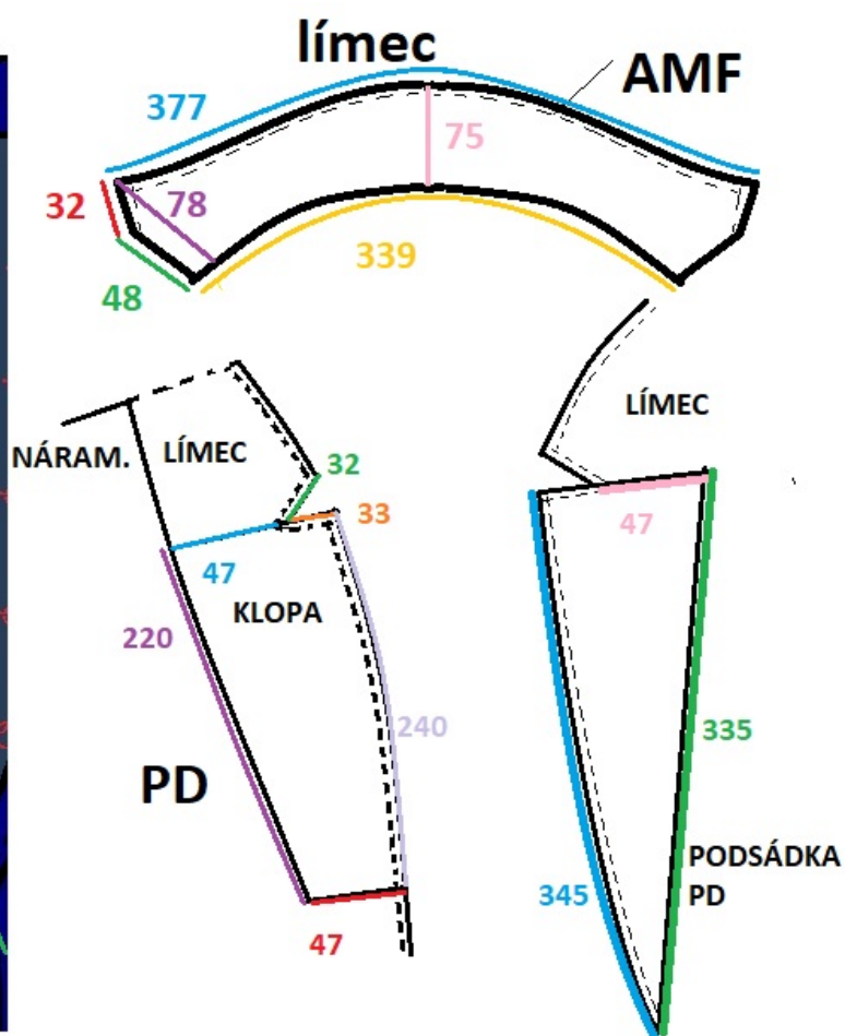
ROZKRES LÍMCE A KLOPY - FAZÓNA
