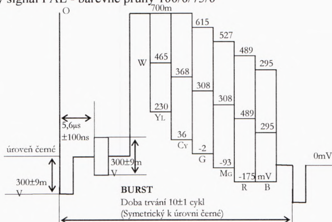
Úplný signál PAL - barevné pruhy 100/0/75/0
