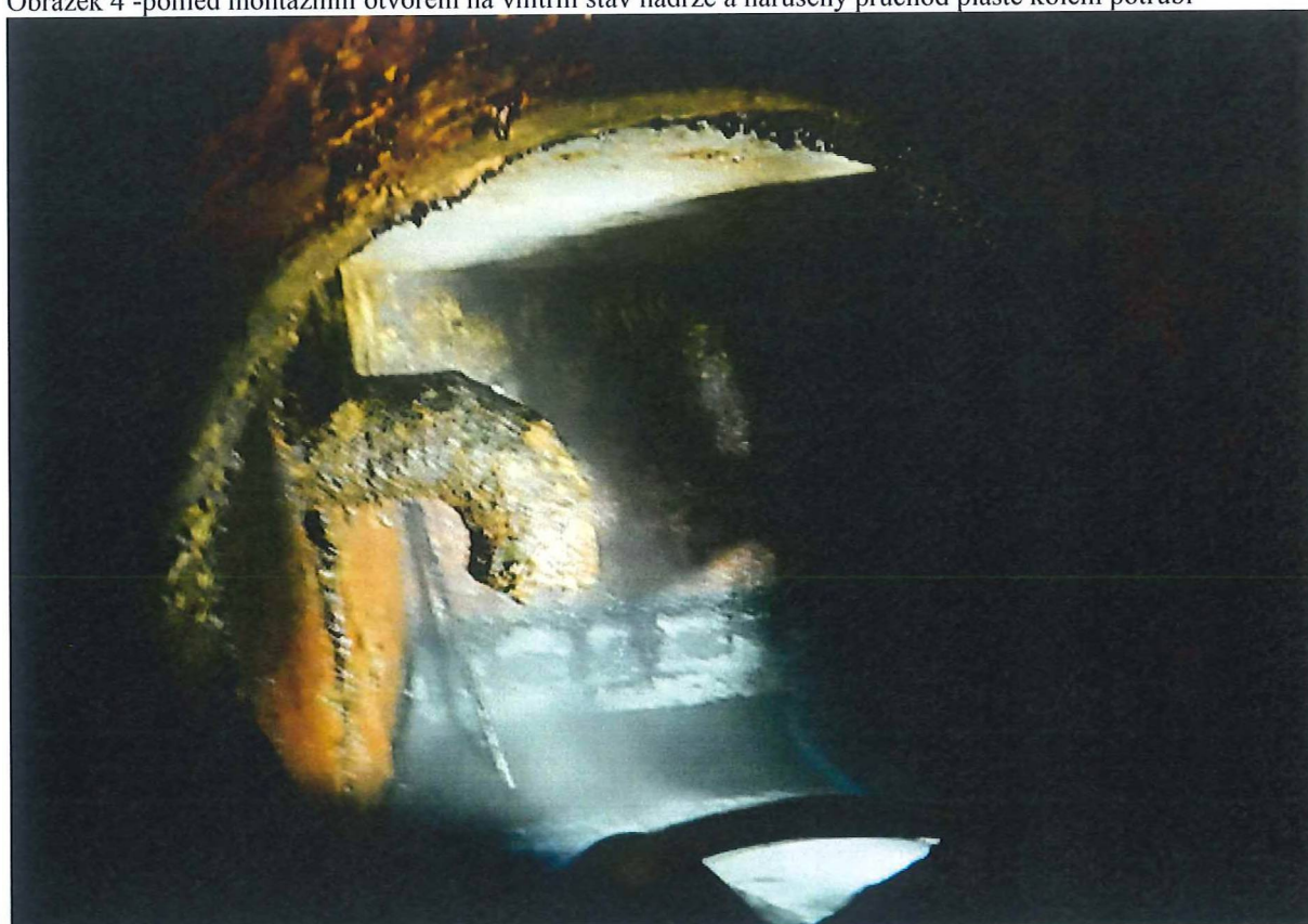
Obrázek 4 -pohled montážním otvorem na vnitřní stav nádrže a narušený průchod pláště kolem potrubí
