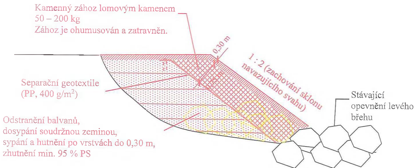
Obr. 2 Odra pod Kozlovem - sanace v místě nátrže.
