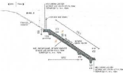
REZ OBSLUŽNEHO SCHODIŠTĚ U OP2 RÍŘIHEŇ 2, 1:100
