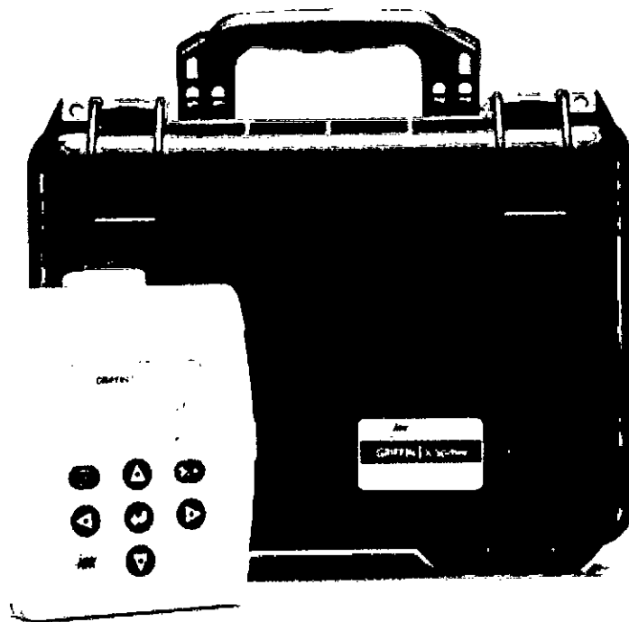
Obrázek č. 2: Mobilní zařízení pro odběr vzorků v hot zóně - X-Sorber
