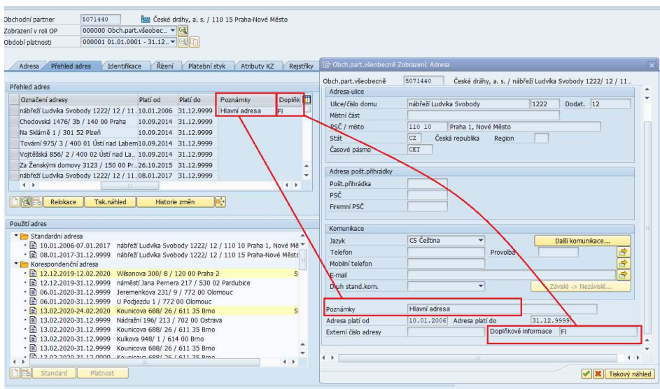
Obrázek 3: Mapping polí z detailní na přehledovou obrazovku
