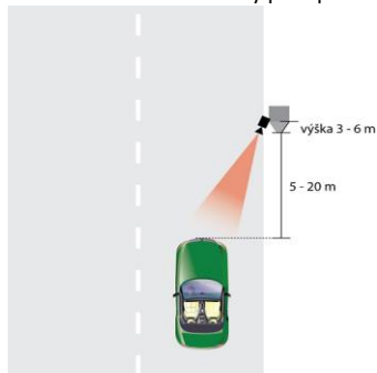
Schéma instalace kamery pro správné rozpoznávání RZ
