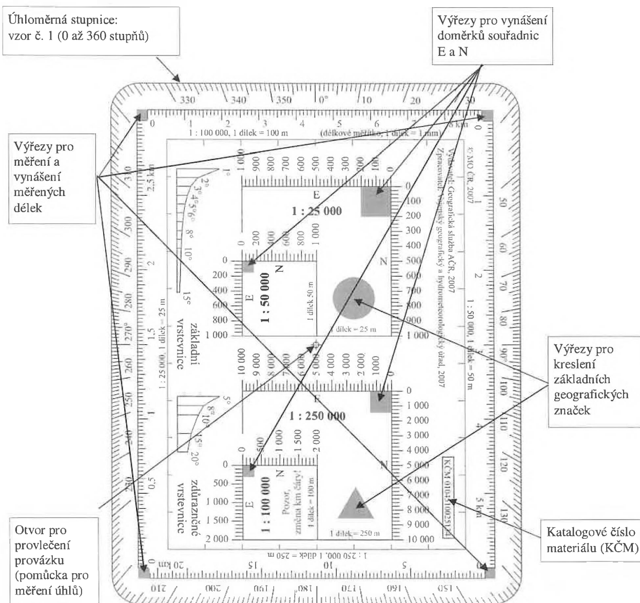
Obrázek 1 Popis Topografické šablony vzoru č. 1
