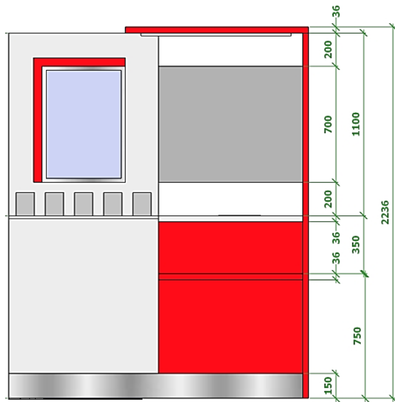
POHLED ČELNÍ:
