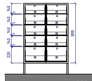
ŘEZ 3-3
