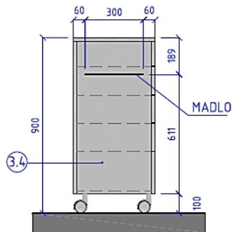
POHLED C
