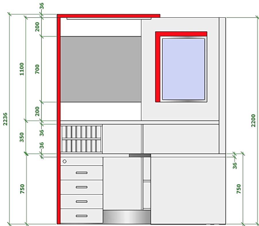
POHLED ZADNÍ:
