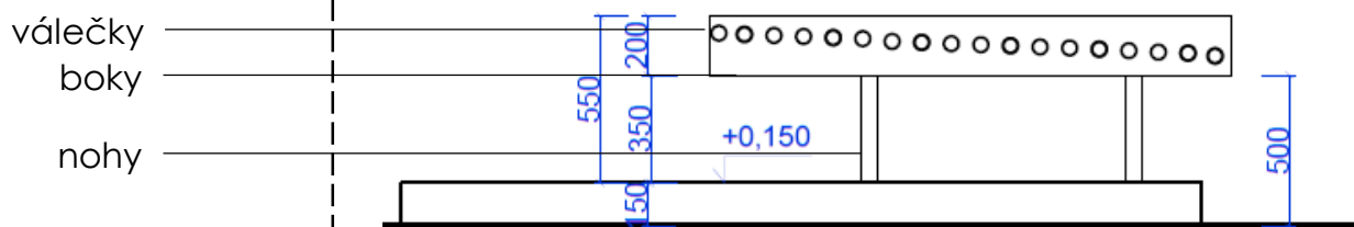
řez podélný
