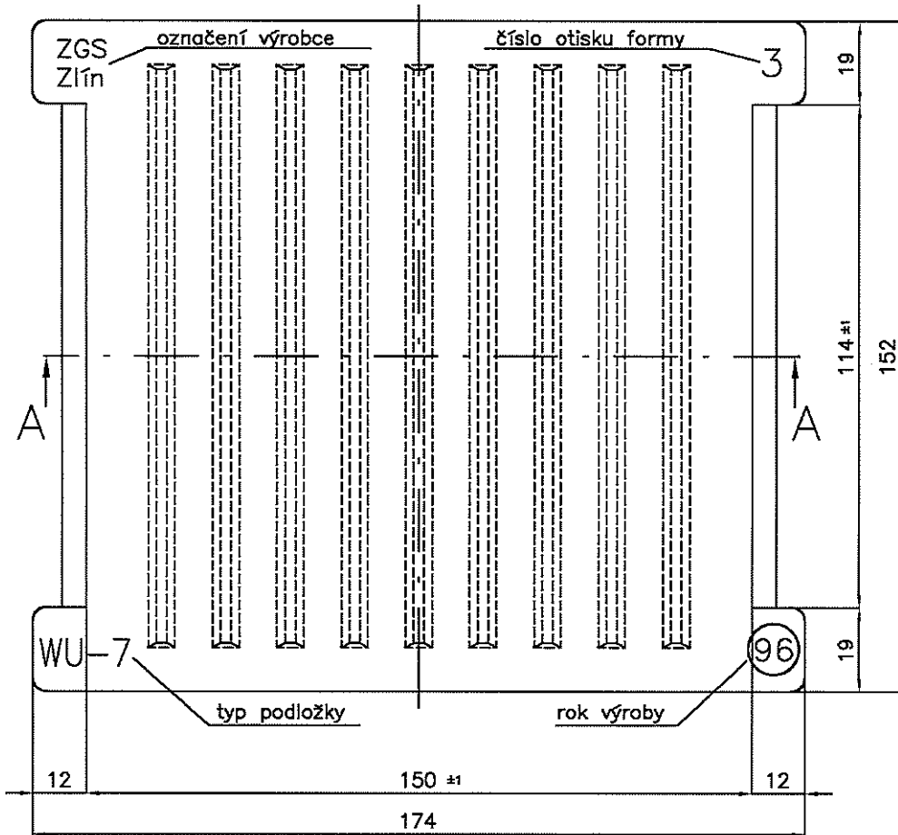
Obr.1 Pohled shora
