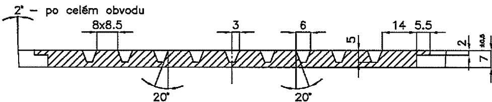
Obr.2 Příčný řez A - A
