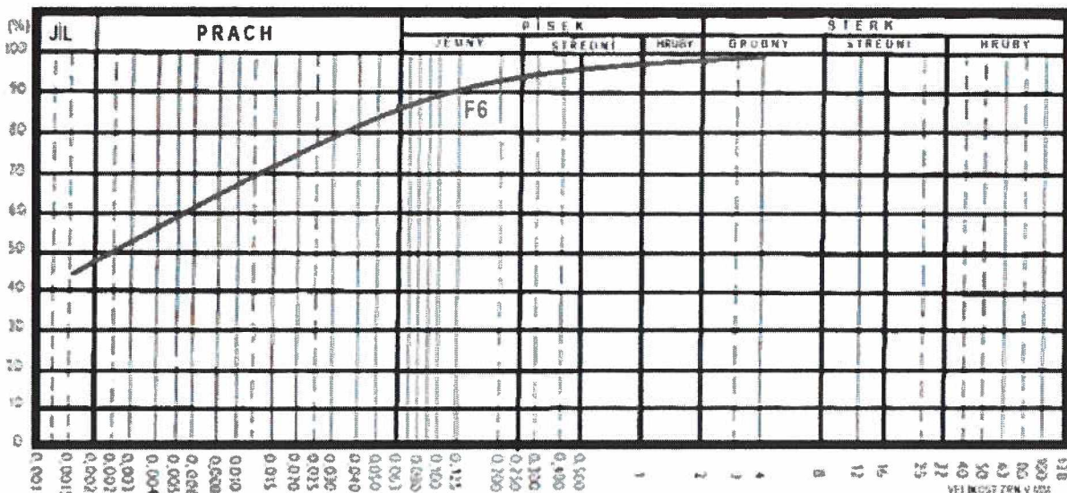
křivky zrnitosti vzorků zeminy – vzorek č. 107 2021
