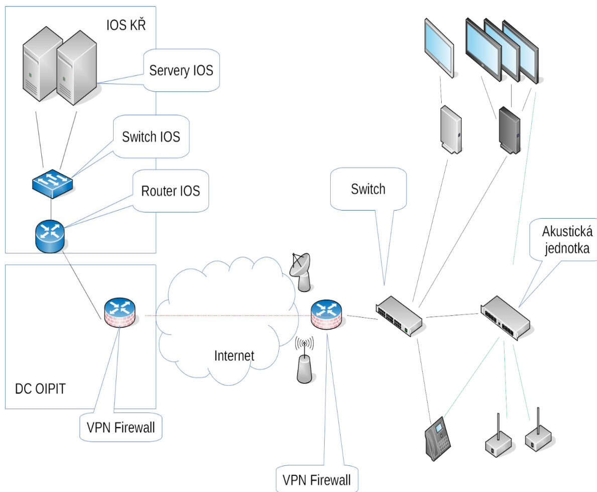
Obr.3 – Navrhované řešení síťového zapojení
