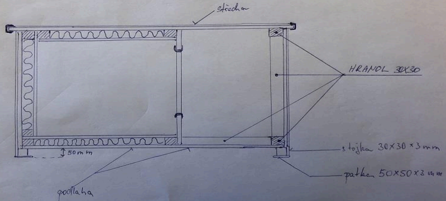
SVISLÝ ŘEZ KONSTRUKCÍ BUDY
