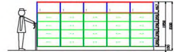
Výškové členění M2-M5
