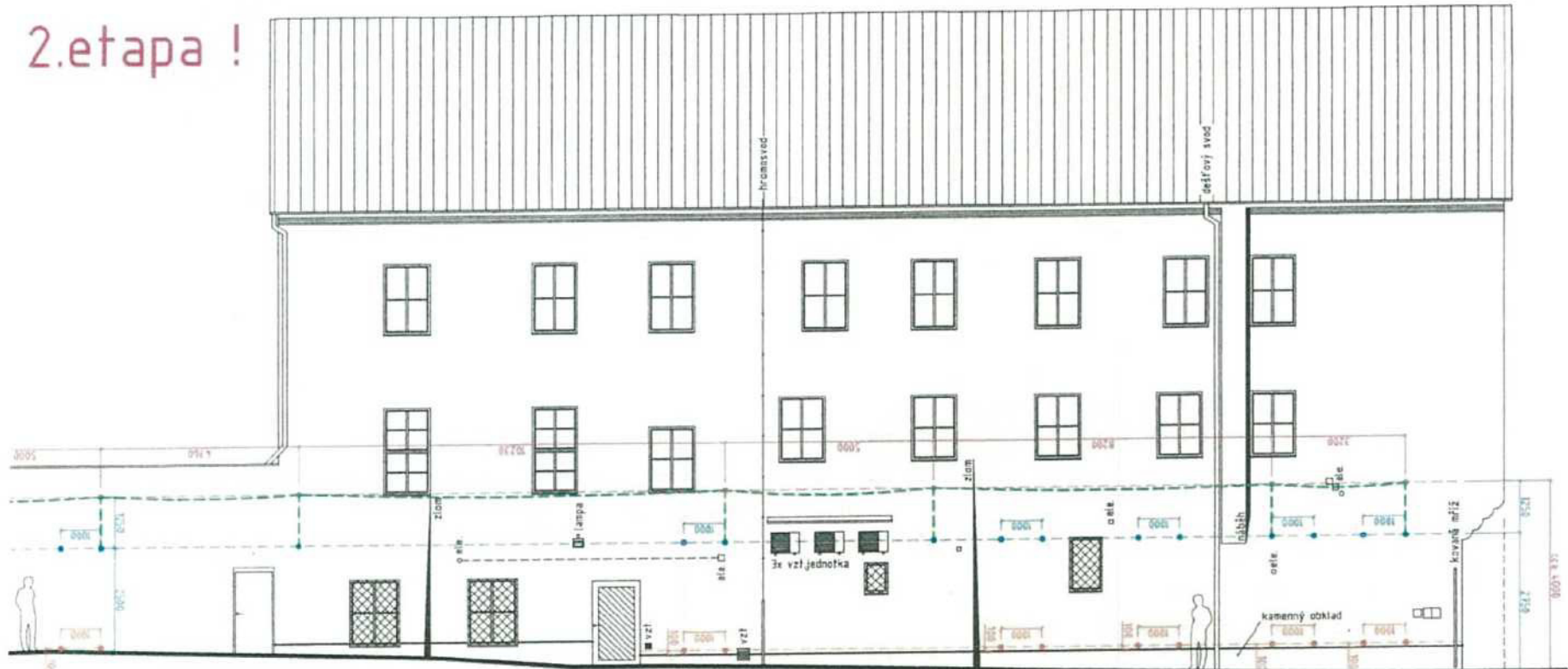
pohled severní
