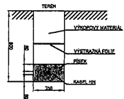
ŘEZ VÝKOPU A-A
