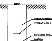
ŘEZ VÝKOPU C-C
