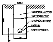
ŘEZ VÝKOPU B-B
