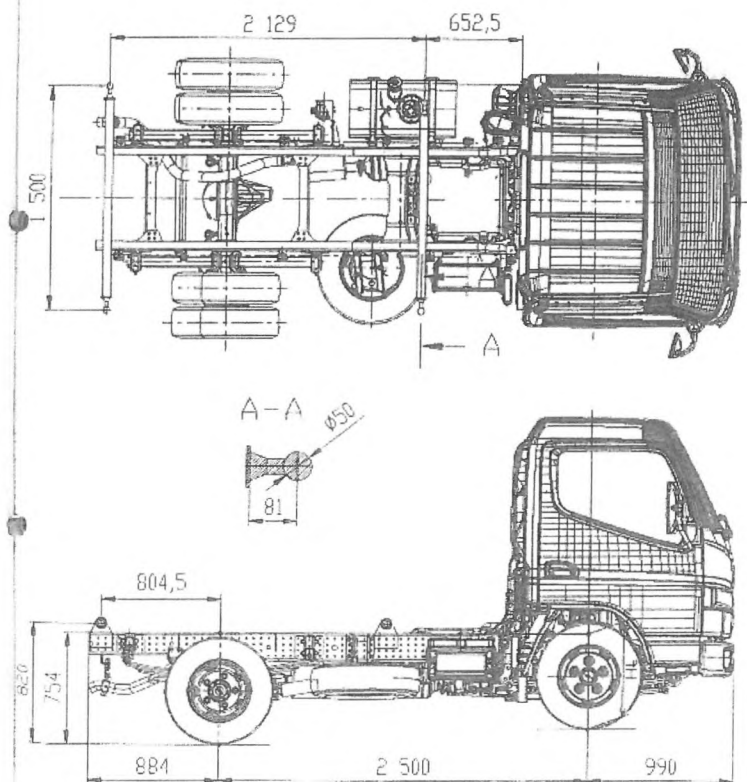
Fuso Canter 6S15 - rozměry nosiče výměrných nástaveb
