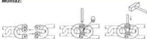
obr.13 – CW spojovací článek
