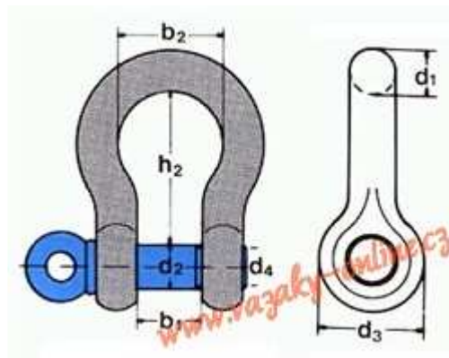
obr.8 – Třmen omega HA2
