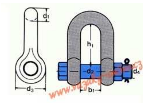
obr.10 – Třmen omega HC1
