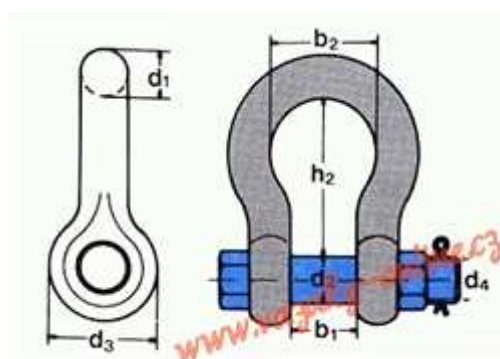
obr.9 – Třmen omega HC2
