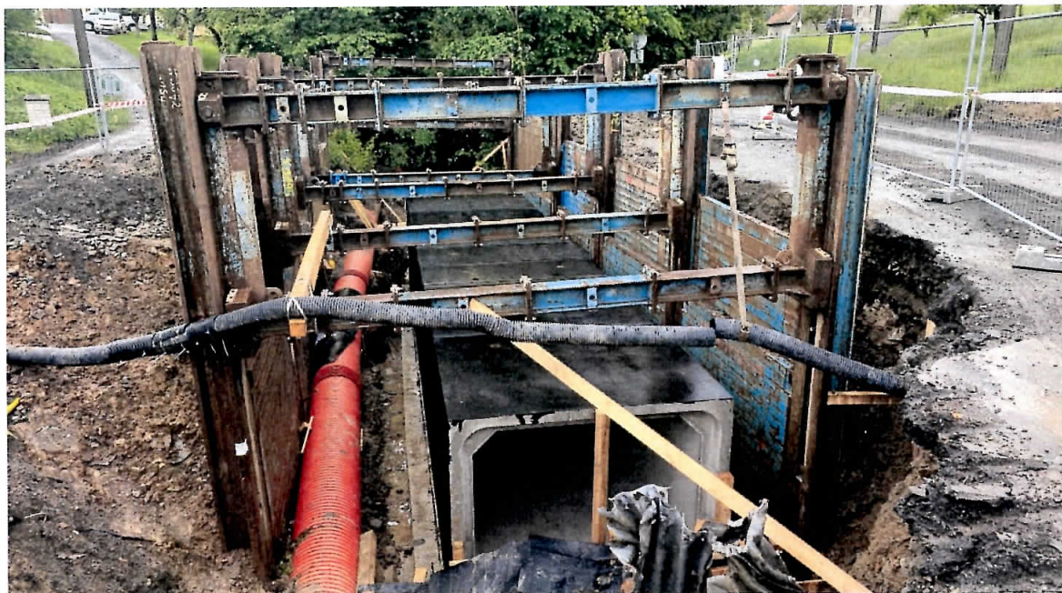
LINEÁRNÍ KLUZNICOVÝ SYSTÉM E+S – STAVBA: MOST EV. Č. 44014-5 PARTUTOVICE
