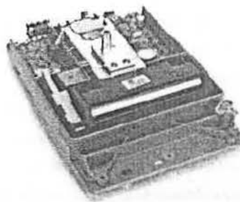
foto monolitického bloku pro uložení vážního systému pro váhy Entris II
