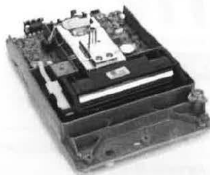
foto monolitického bloku s uložením vážního systému pro váhy Entris II
