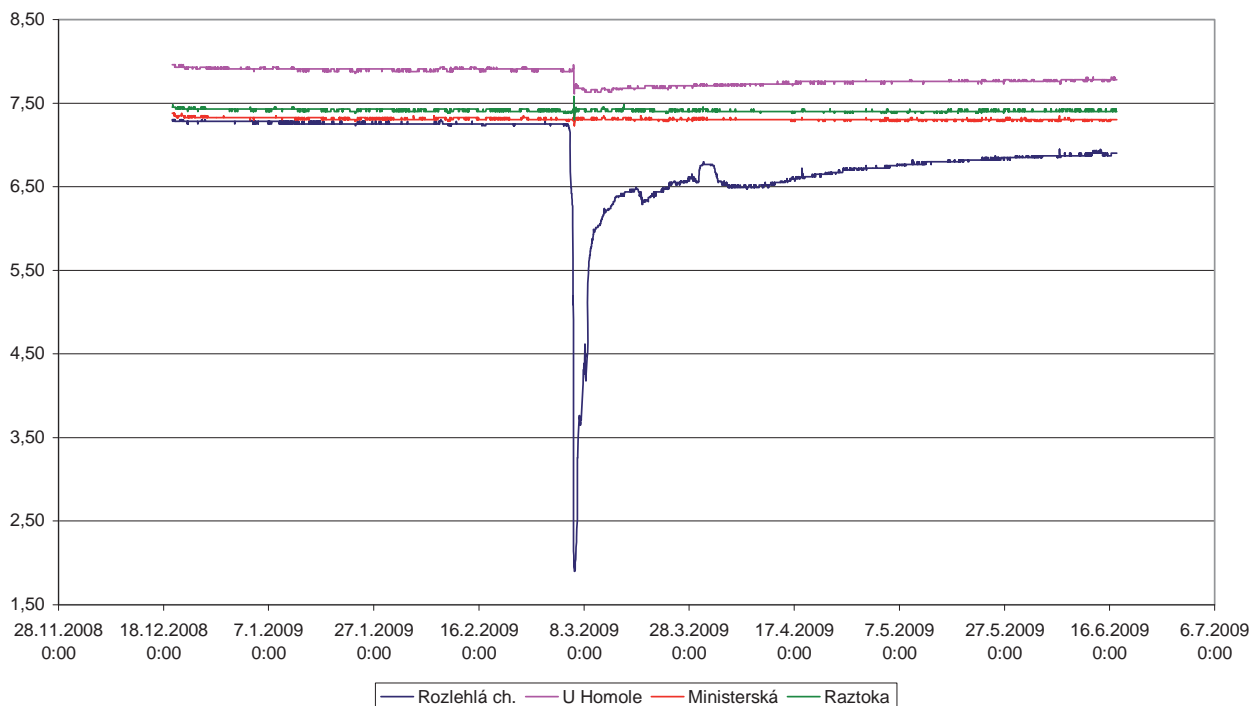
Obr. 9 Ovlivnění teploty vzduchu v Amatérské jeskyni kolísáním hladiny podzemního toku.
