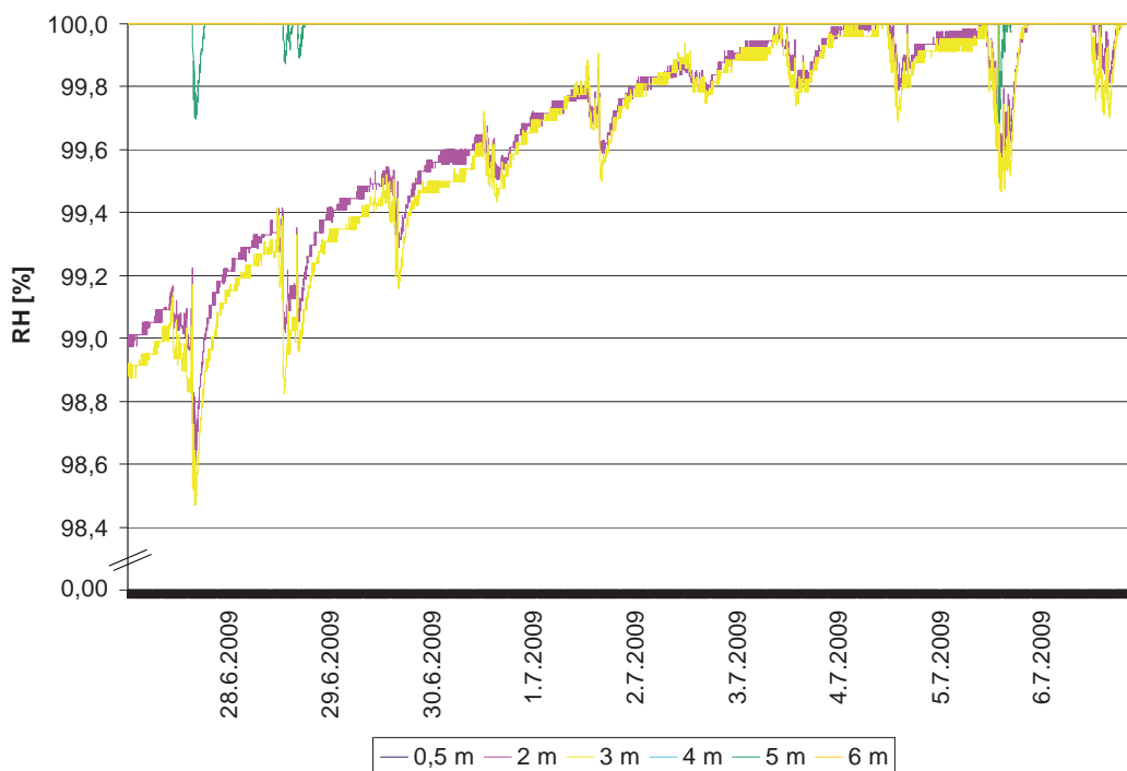
Obr. 20 Vlhkost vzduchu v Kateřinské jeskyni (27. 6. - 6. 7. 2009) – vertikální profil.
