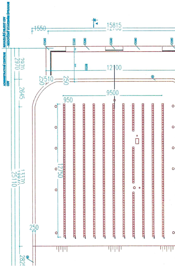
Obr.2. Půdorys kotevní plán – dodatečné bodové kotvení
