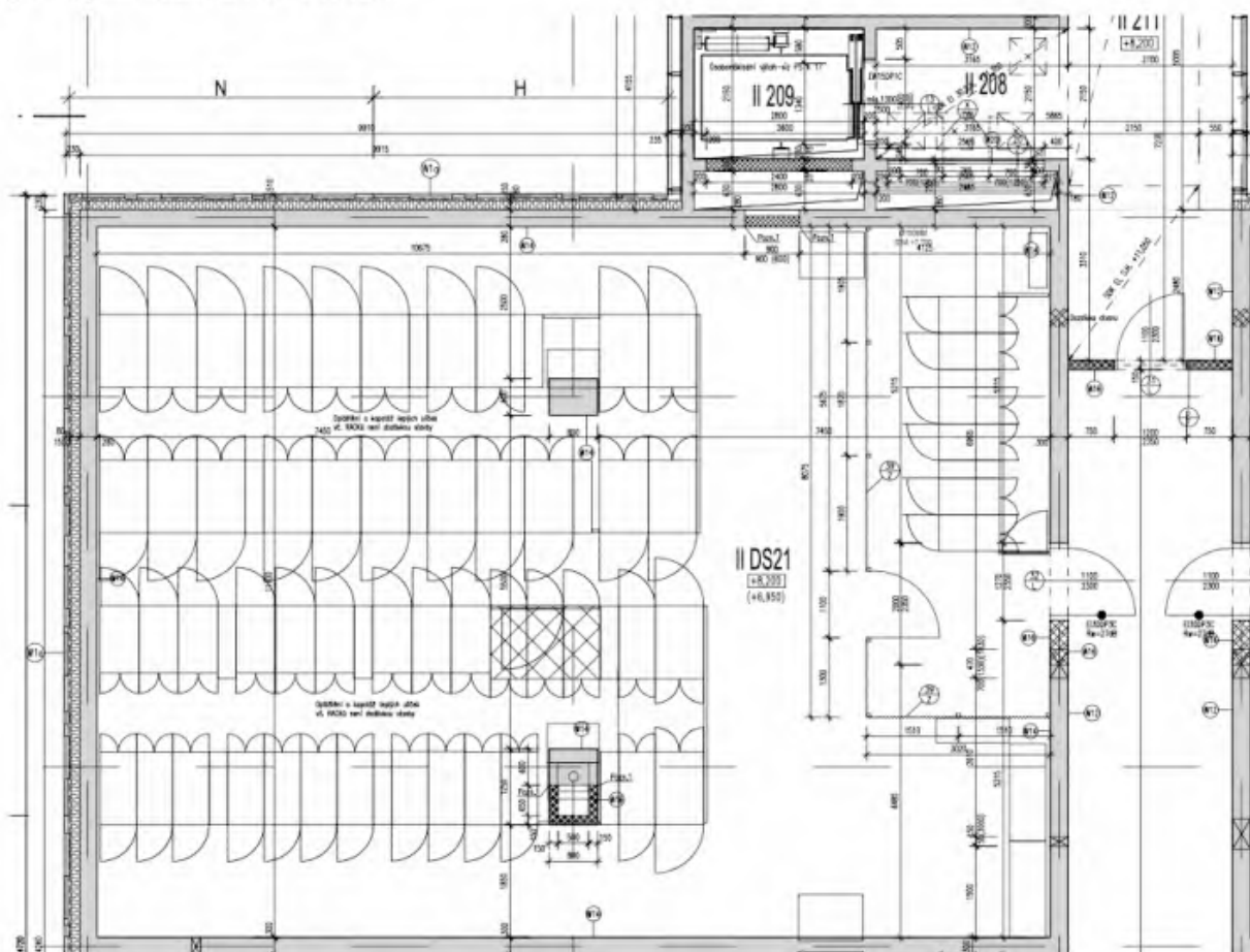
Obrázek: Půdorys datového sálu
