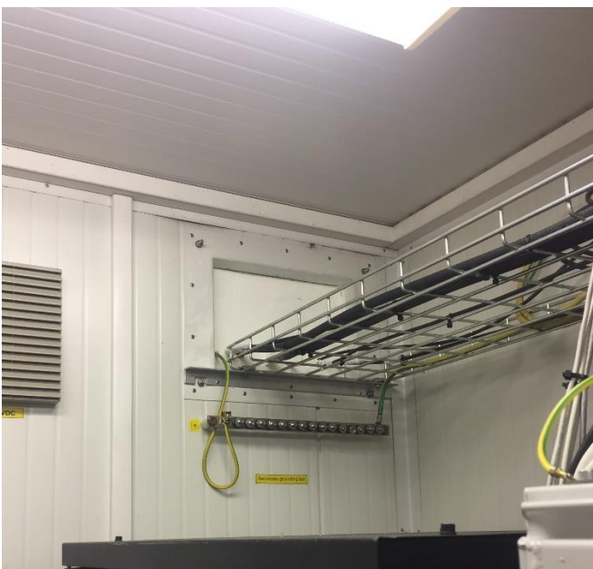
Obr. 5 Výstup anténních svodů z kontejneru
