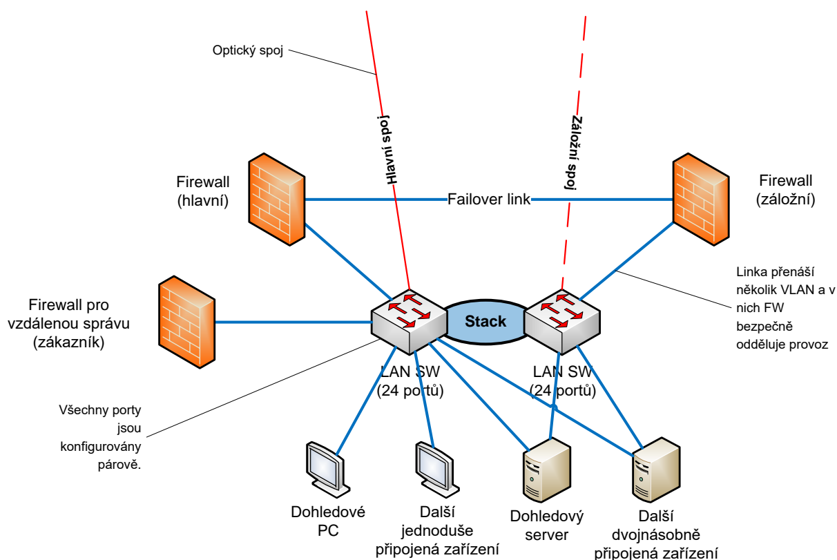
Obrázek 1: Fyzické zapojení
