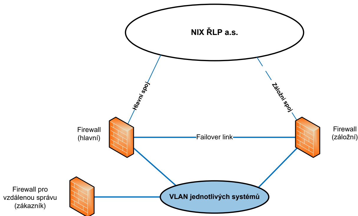
Obrázek 2: Logické zapojení
