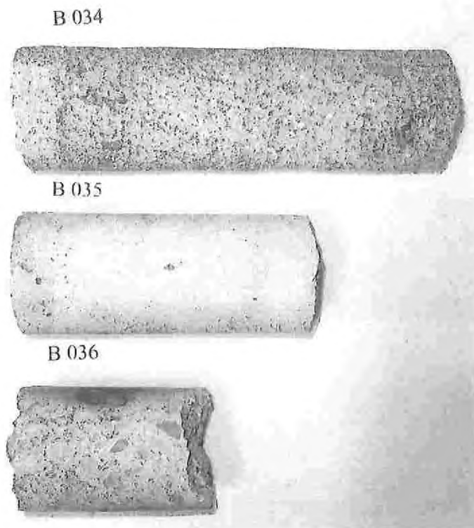
Obr. 3.: Vývrtý z betonu nosné konstrukce po dodání do laboratoře - druhá skupina
