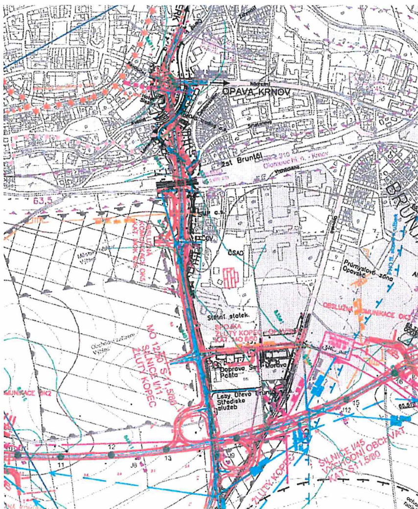
Obrázek 1: Přehledná situace přeložky silnice I/11 Bruntál – Žlutý kopec
