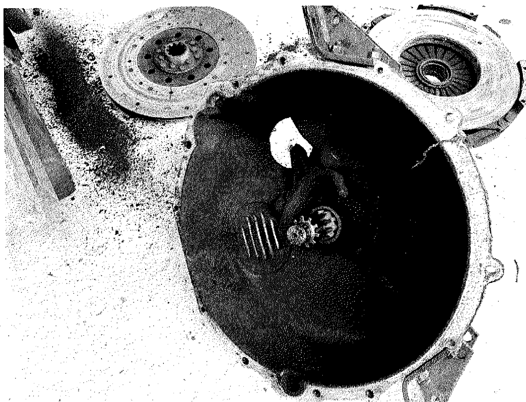
Přidřená a opotřebená vidlice spojky
