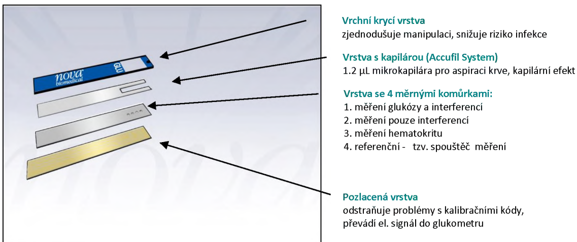
Obr. 1: Technologie MultiWell™ - unikátní koncepce testovacího stripu: 4 vrstvy, 4 měřné komůrky
