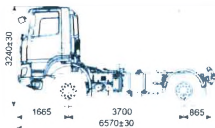
Výškové rozměry platí pro zatížené vozidlo
