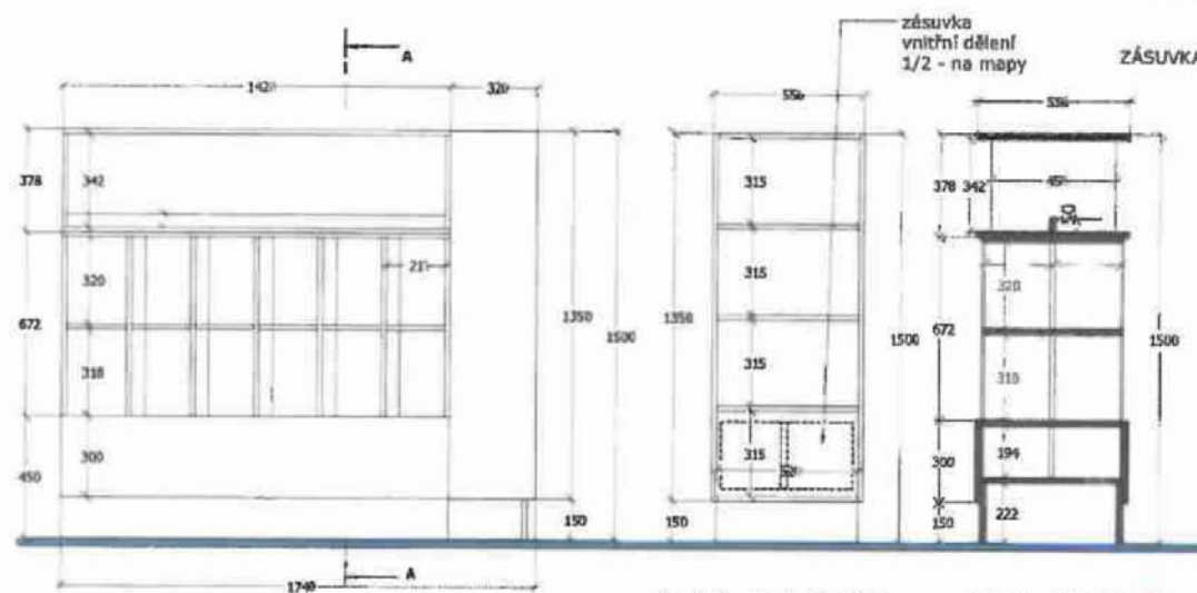
čelní pohled M 1:20
