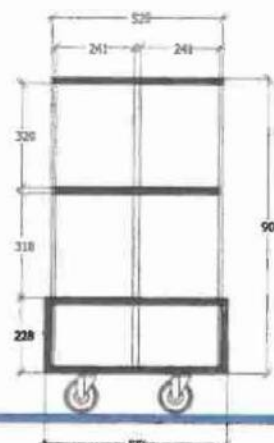
bokořez M 1:15
