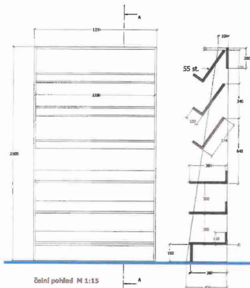
bokořez AA M 1:15
