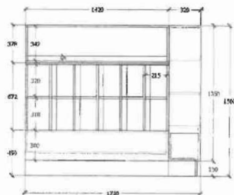
čelní pohled M 1:20
