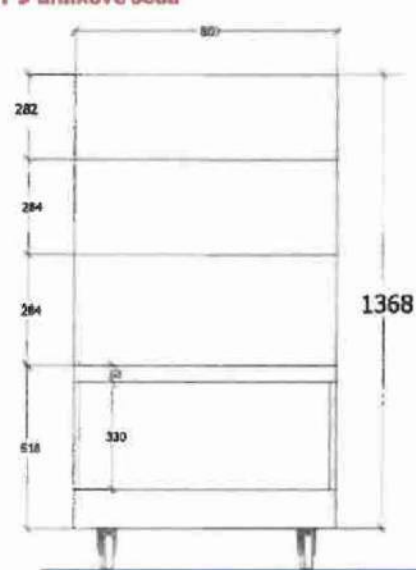
čelní pohled M 1:15
