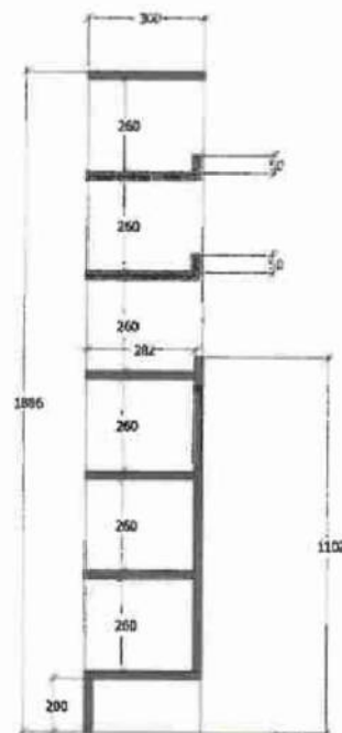
bokořez AA M 1:15
