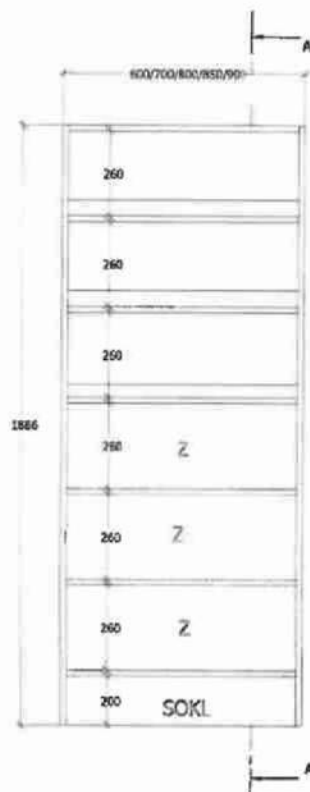
čelní pohled M 1:15
