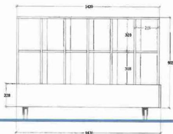
čelní pohled M 1:15
