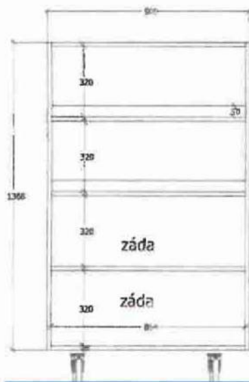
čelní pohled M 1:15
