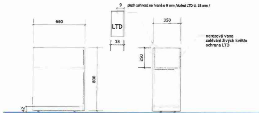
čelní pohled M 1:15
