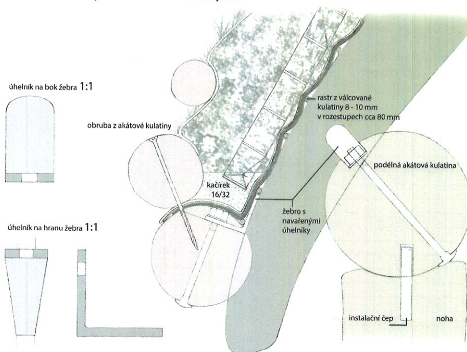
detail kotvení nohy do žebra a detail obruby 1:2
