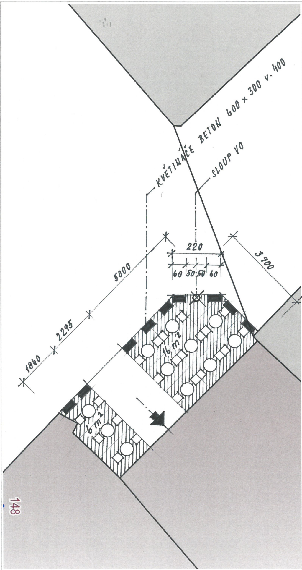
SITUAČNÍ SCHÉMA 1 : 100 ZAHRAĎKA CORSO
