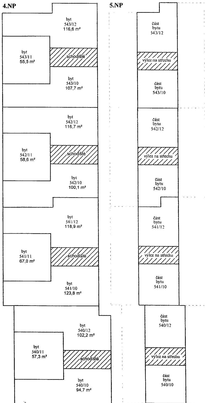
Schema budovy: Husova č.p. 540, 541, 542 a 543 , obec Náměšť nad Oslavou, část obce Náměšť nad Oslavou
